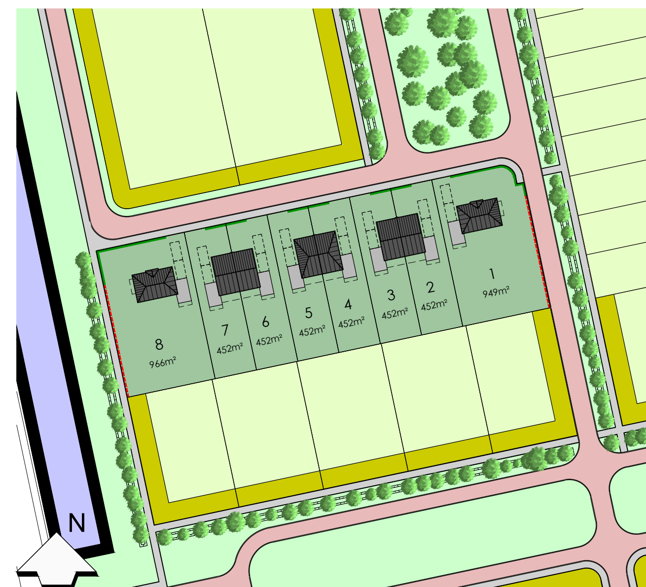
Renvooi — Metalen hekwerk +1800mm met hedera — Haag +1000mm Schaal 1:1000
