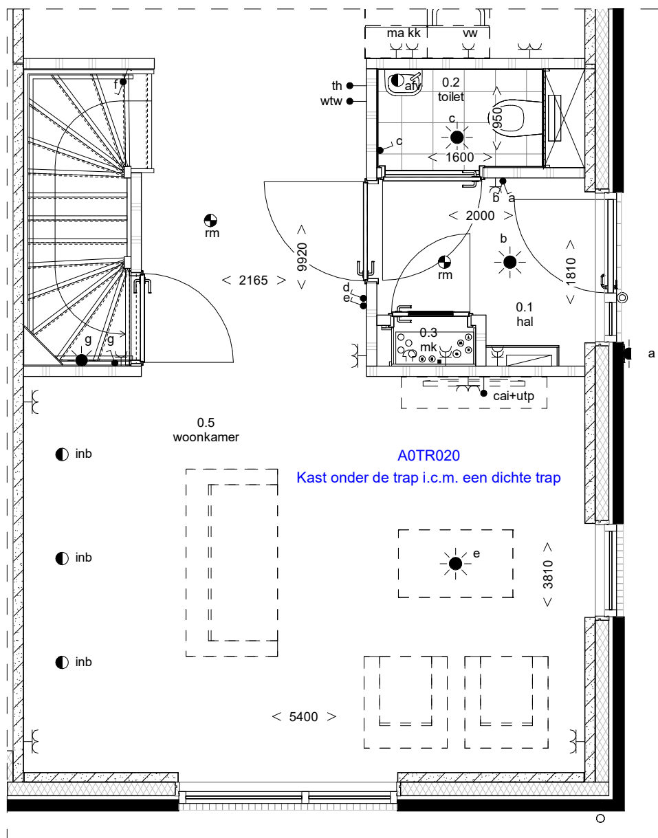
begane grond 1 : 50
