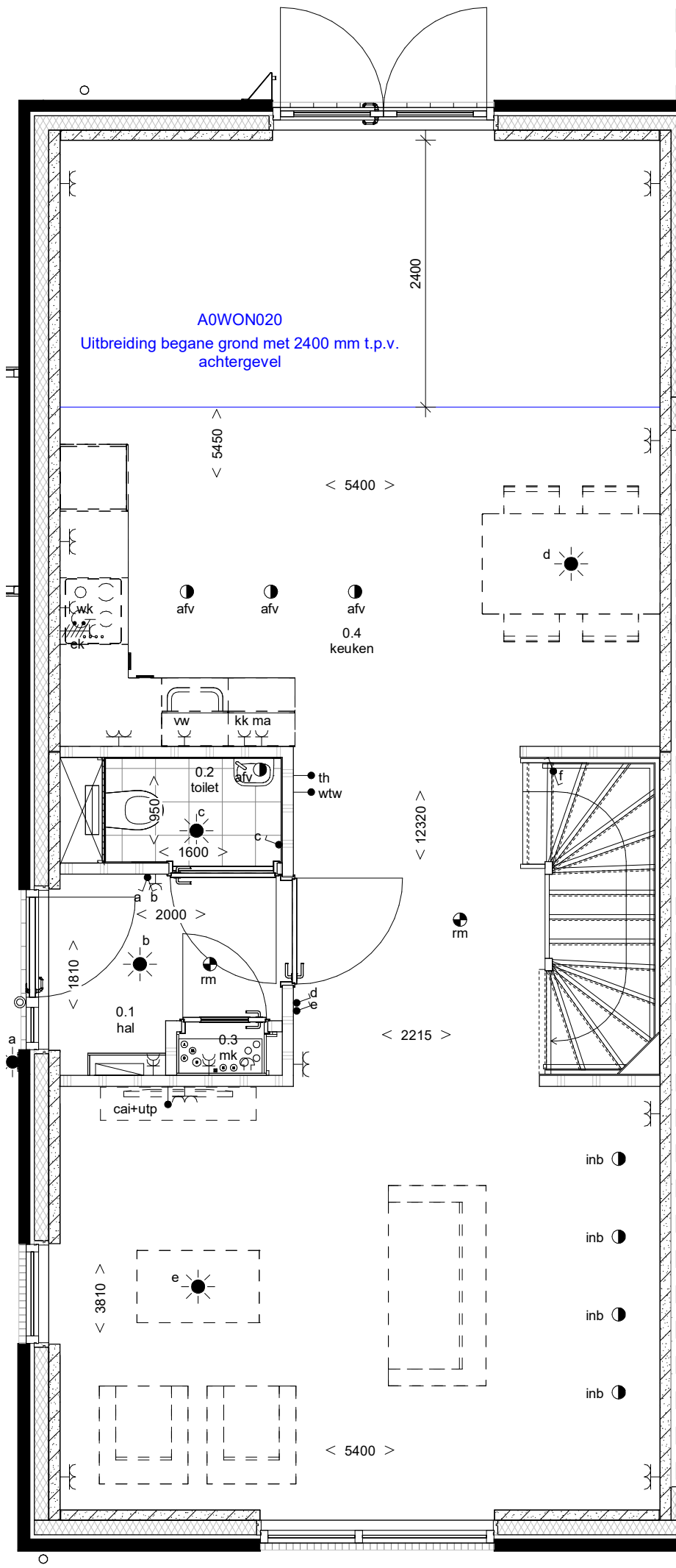
begane grond 1 : 50
