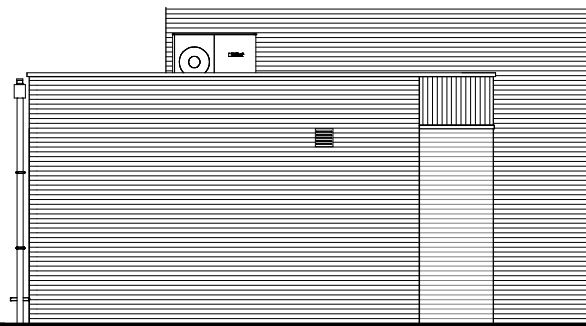
linkerzijgevel 1 : 100
