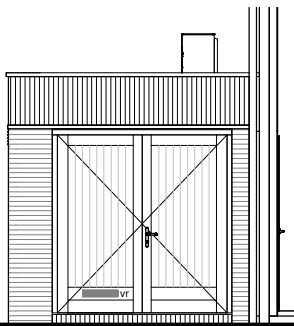
voorgevel 1 : 100
