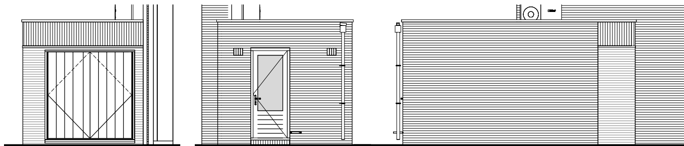
voorgevel 1 : 100
