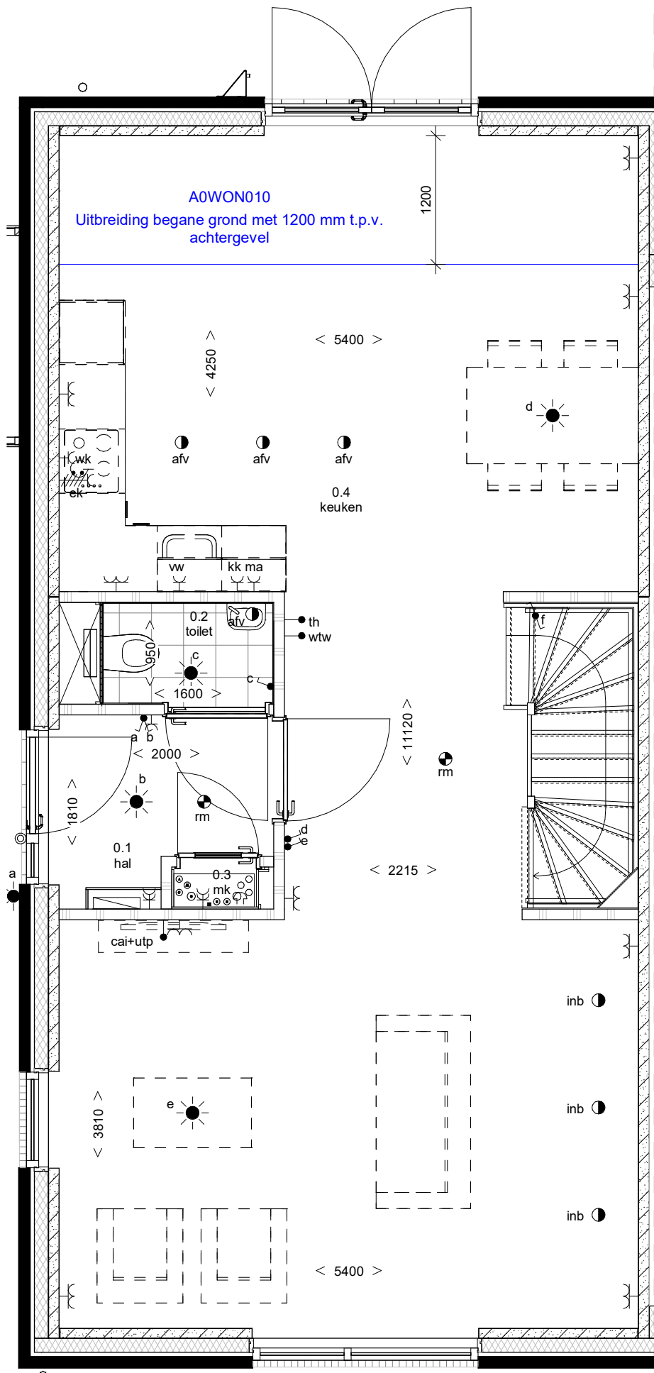
begane grond 1 : 50
