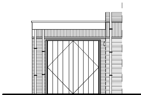
voorgevel 1 : 100
