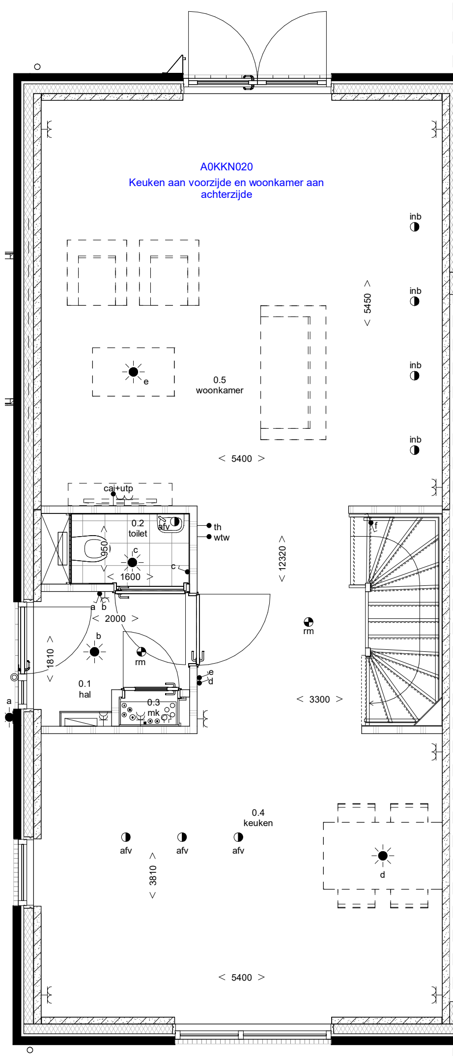
begane grond 1 : 50
